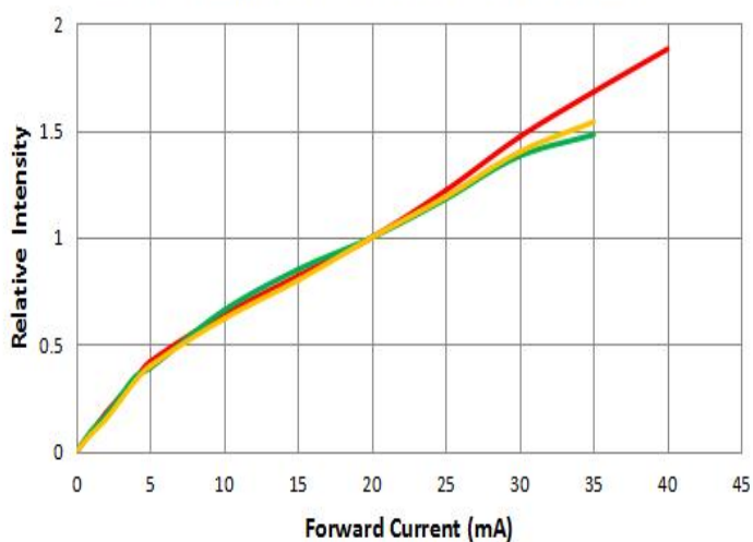
相对光强与电流特性曲线
