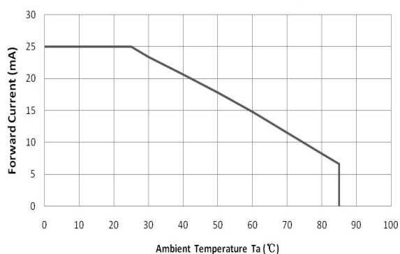
最大正向电流与环境温度特性曲线
