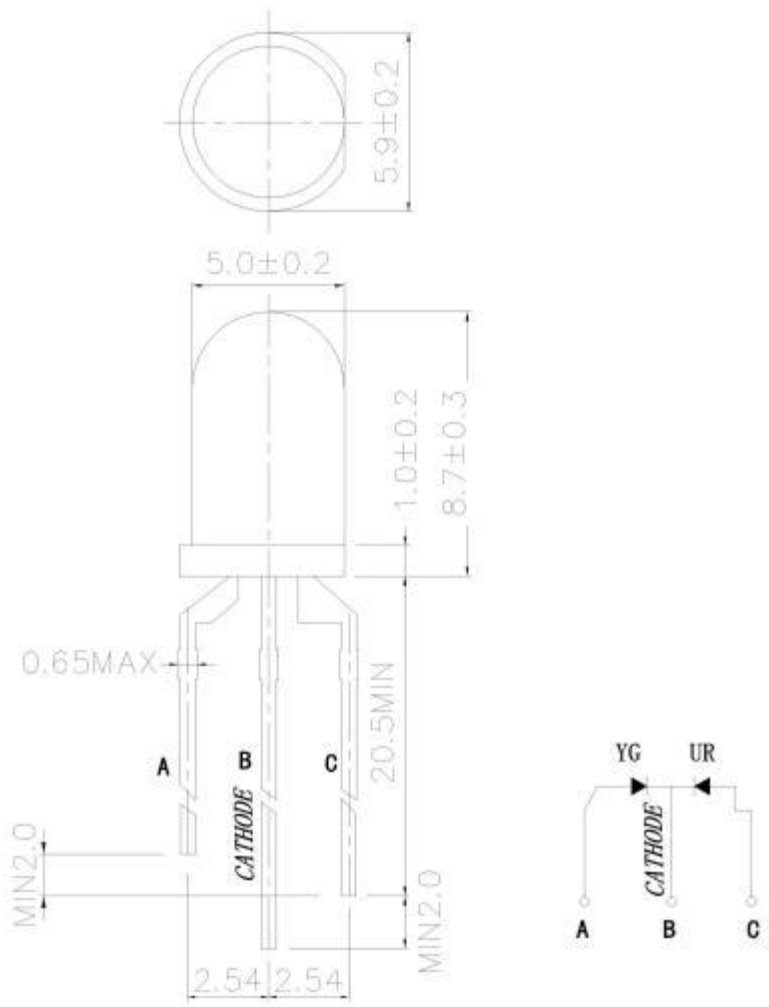
外形图 Outline dimensions:
