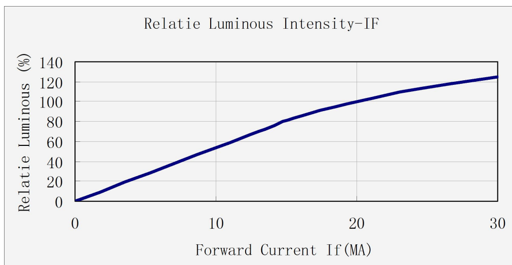
相对发光强度与正向电流关系图:
