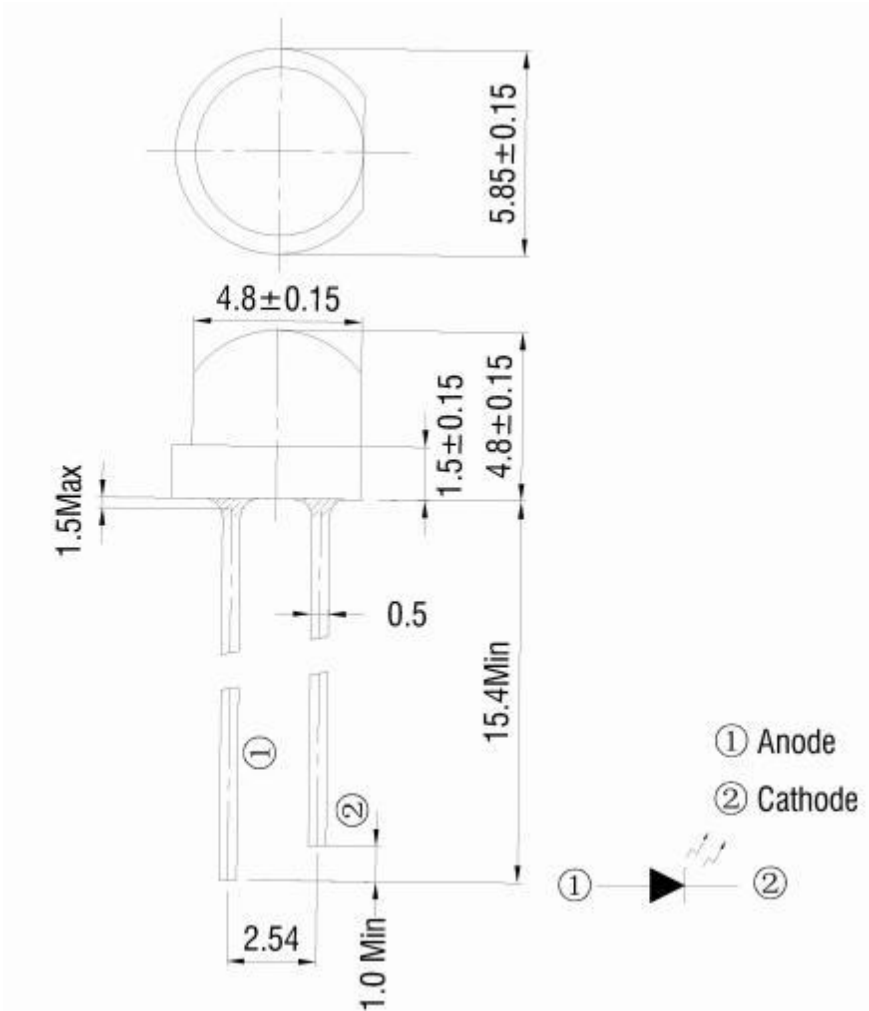
外形图 Outline dimensions: （单位：mm）
