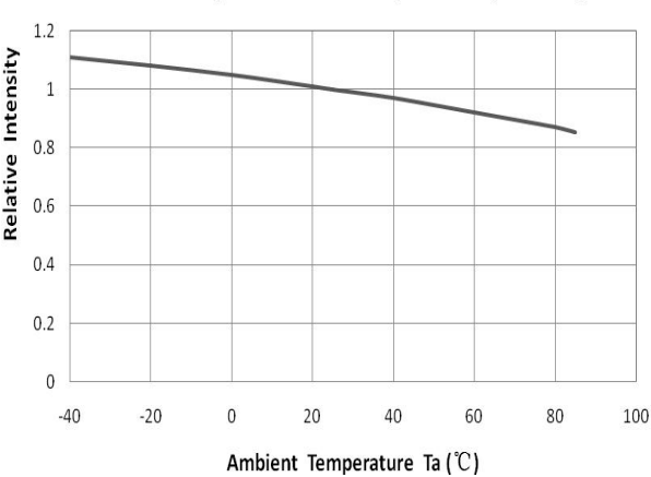
相对光强与环境温度特性曲线 Relative Intensity VS. Ambient Temperature (Ta=25℃)
