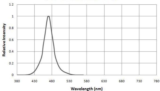
光谱分布特性曲线 Spectrum Distribution (Ta=25℃)
