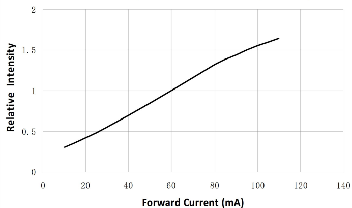
相对光强与电流特性曲线 Relative Intensity VS. Forward Current (Ta=25℃)
