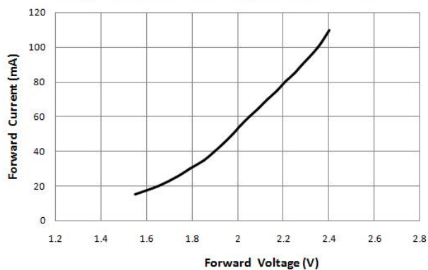
伏安特性曲线
