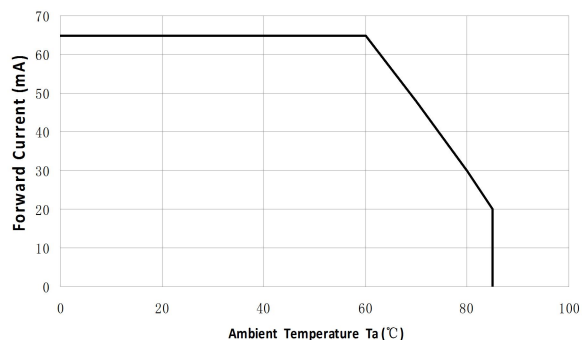
最大正向电流与环境温度特性曲线
